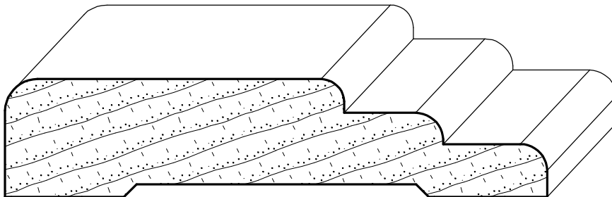
IH-1412 7/8" x 4"
