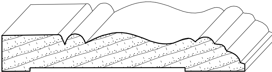
IH-472 1 1/16" x 4-5/16"
