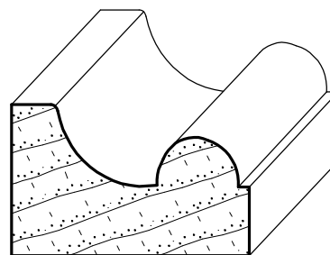
IH-228 7/8" x 1-3/8"
