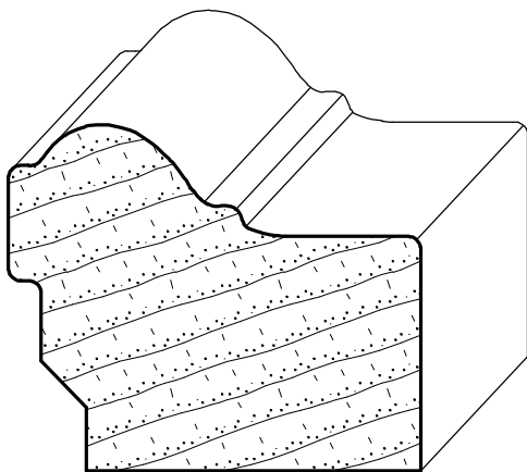
IH-100 1-11/16" x 2"
