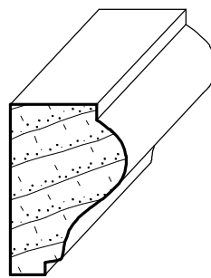
IH-185 11/16" x 1"
